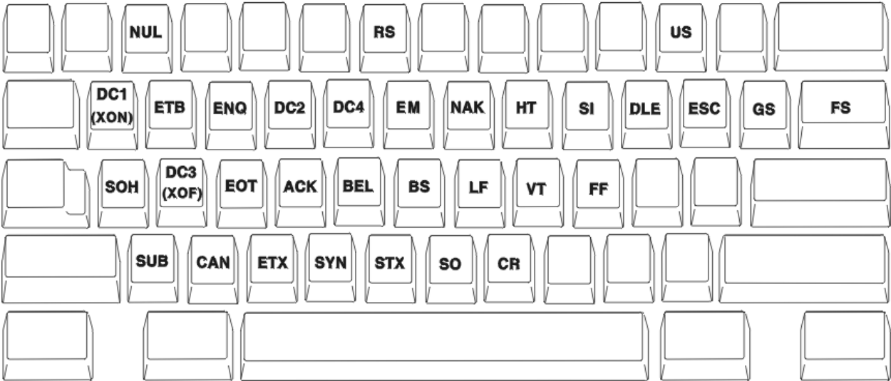
Figure 8. Carte des codes de contrôle du segment principal du clavier pour le clavier américain amélioré on page 2
