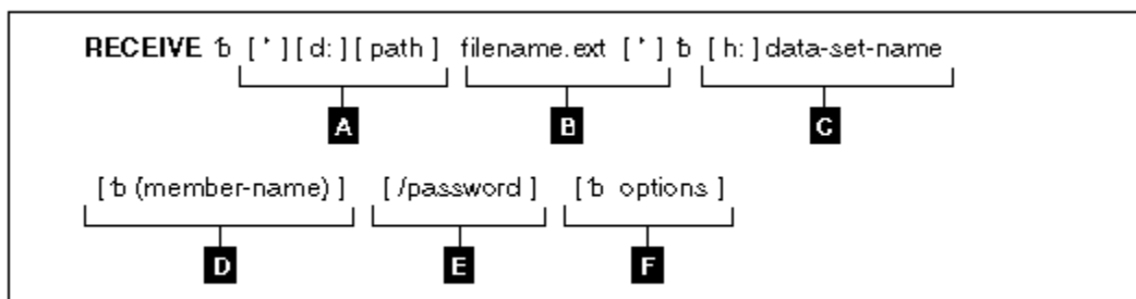
图 4. MVS/TSO RECEIVE 命令语法
