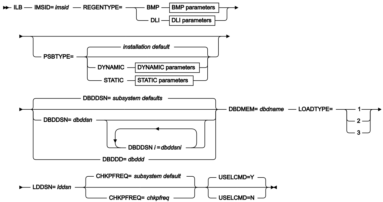
図 145. Syntax
