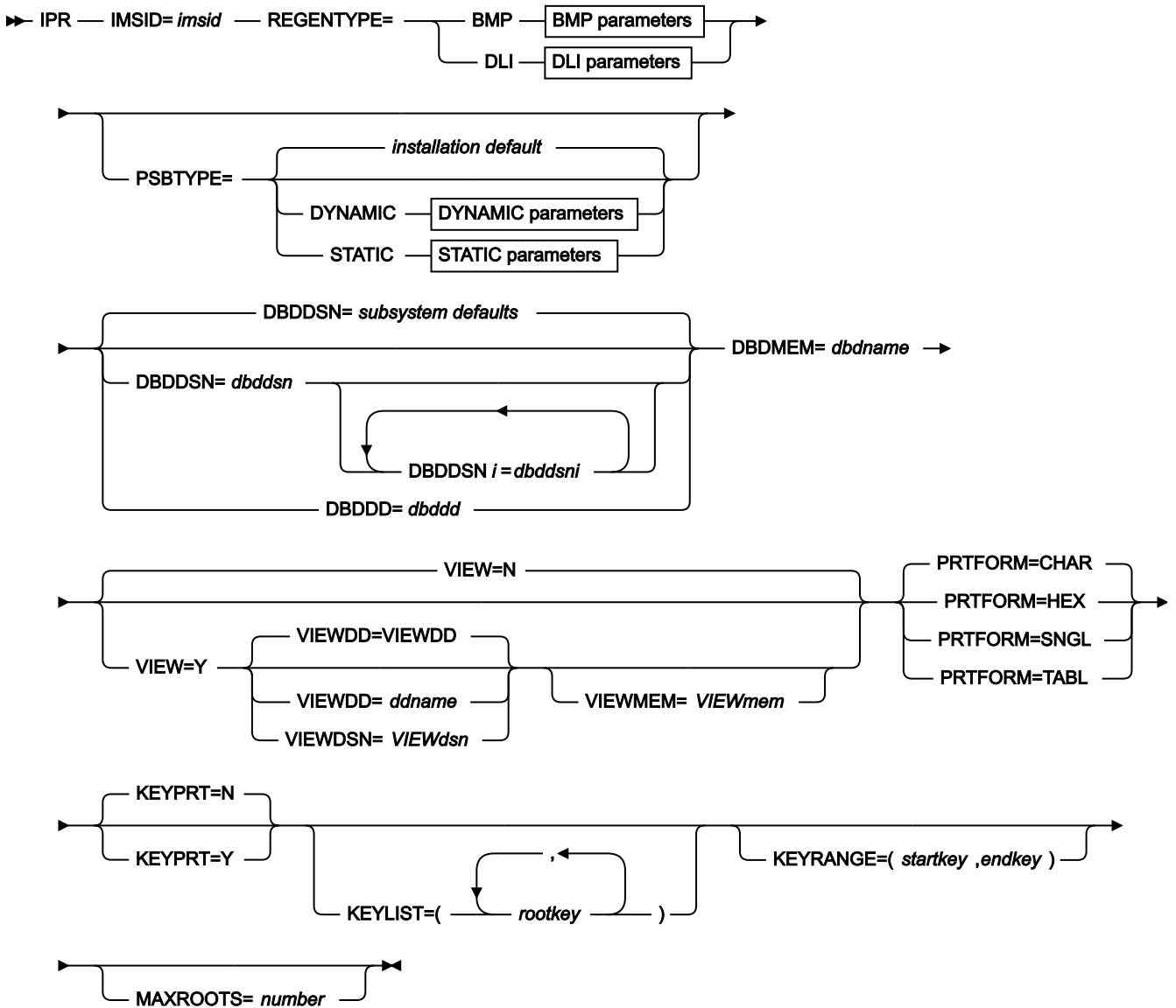
図 150. Syntax
