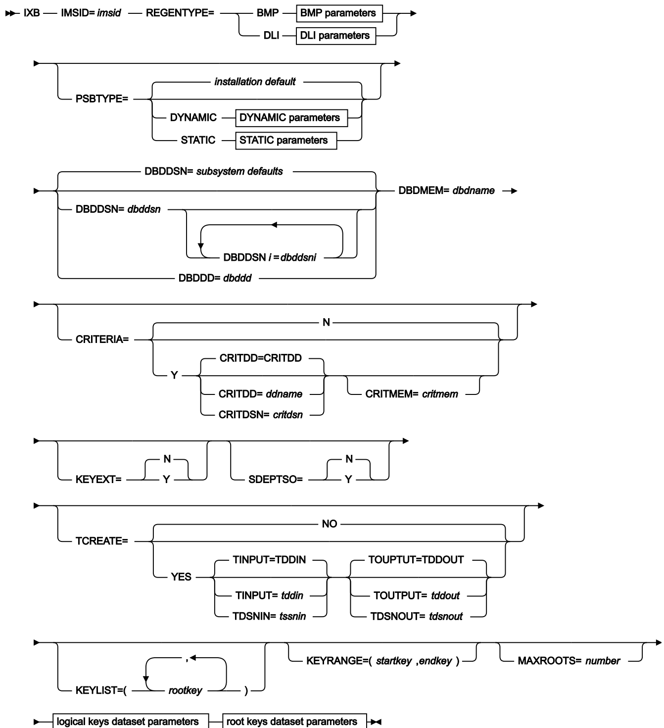
図 141. Syntax
