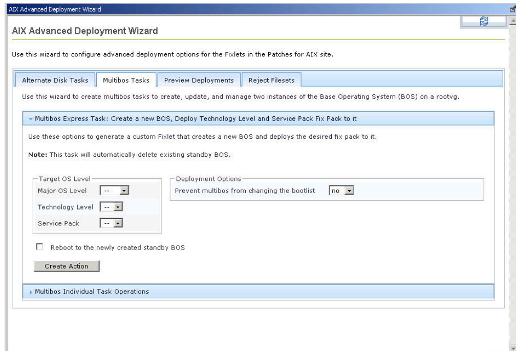
図 28. multibos 高速タスク
