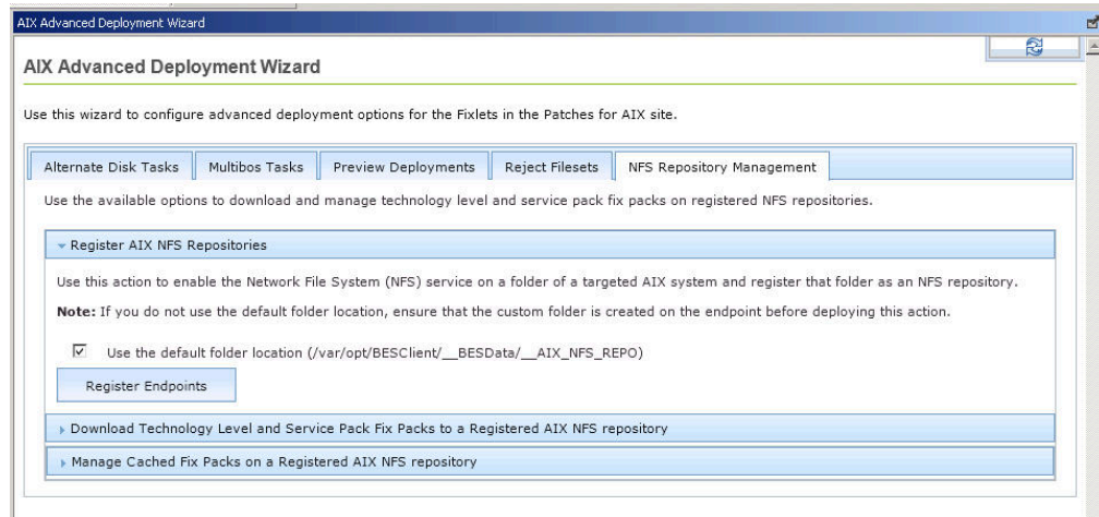
図 34. AIX NFS リポジトリの登録
