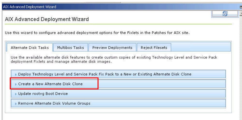
図 22. 新規代替ディスク・クローンの作成
